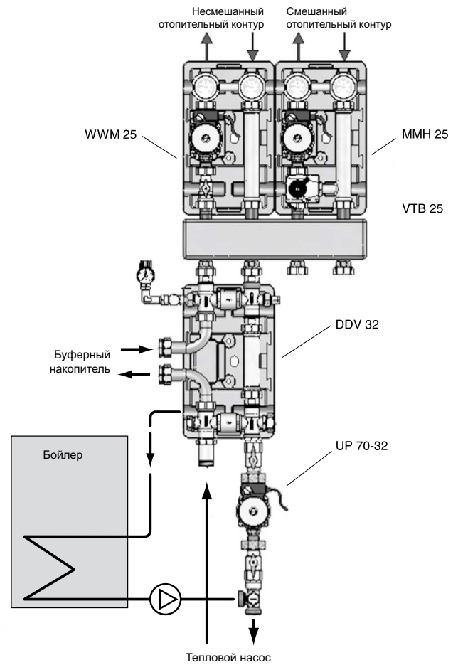
Рис. 8.7: Обвязка двойного распределителя без перепада давления для режима отопления и приготовления горячей воды
