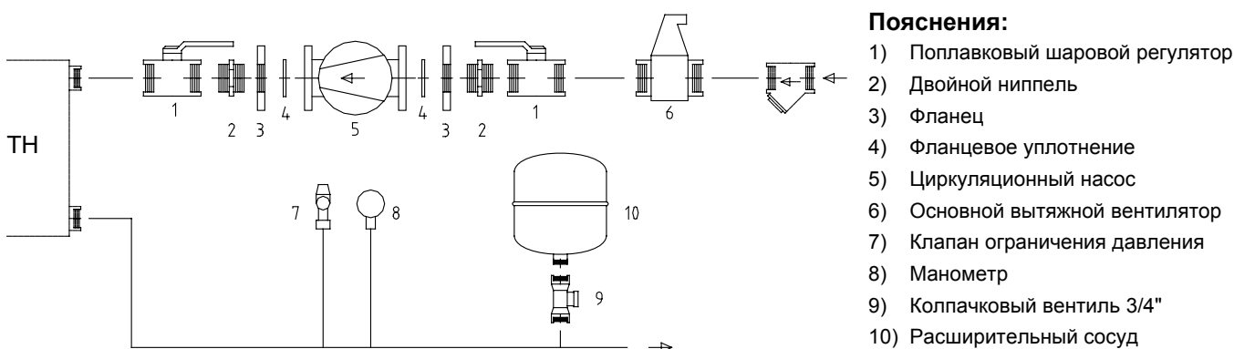
Рис. 3.5: Структура трубопровода соляного раствора, вкл. встроенные компоненты
